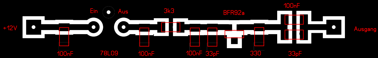
Rauschgenerator SMD
